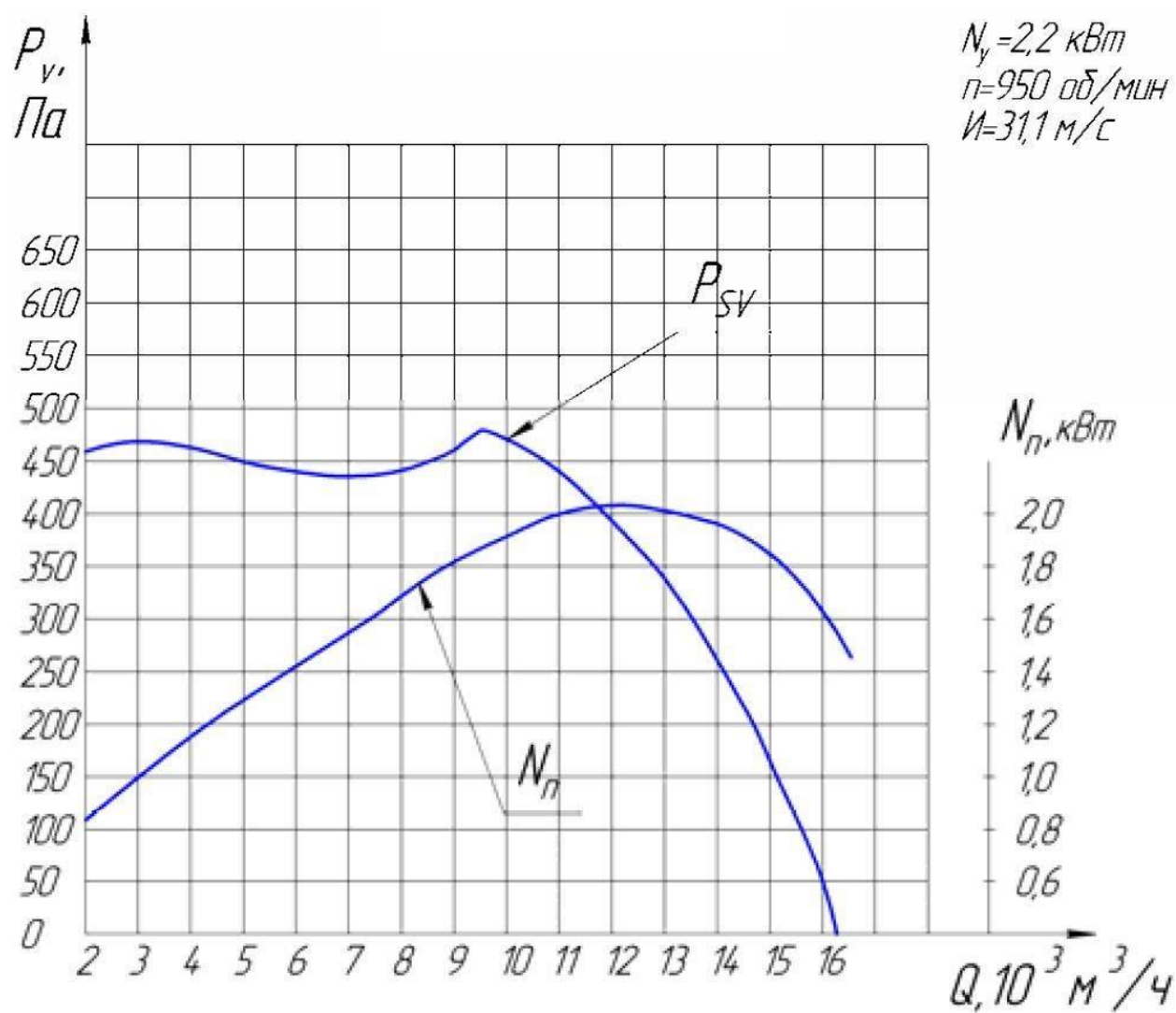
Вентилятор ВКР-6,3
