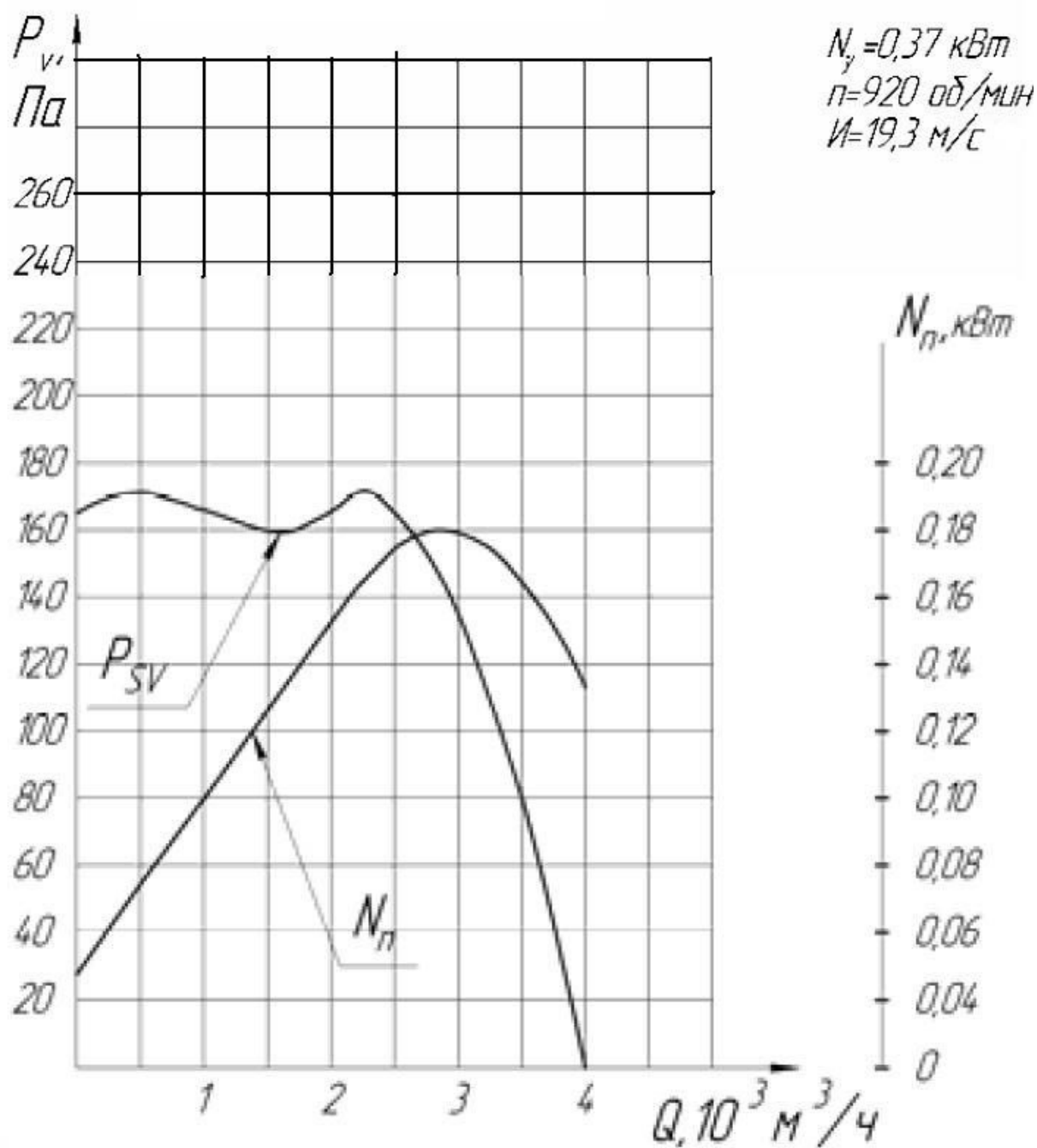
Вентилятор крышный ВКР-4
