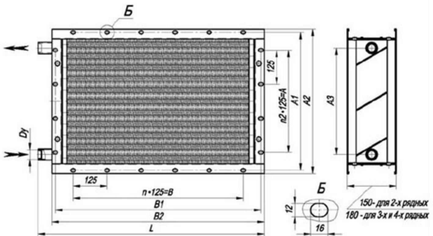
Рисунок 4-5 Размеры, мм
