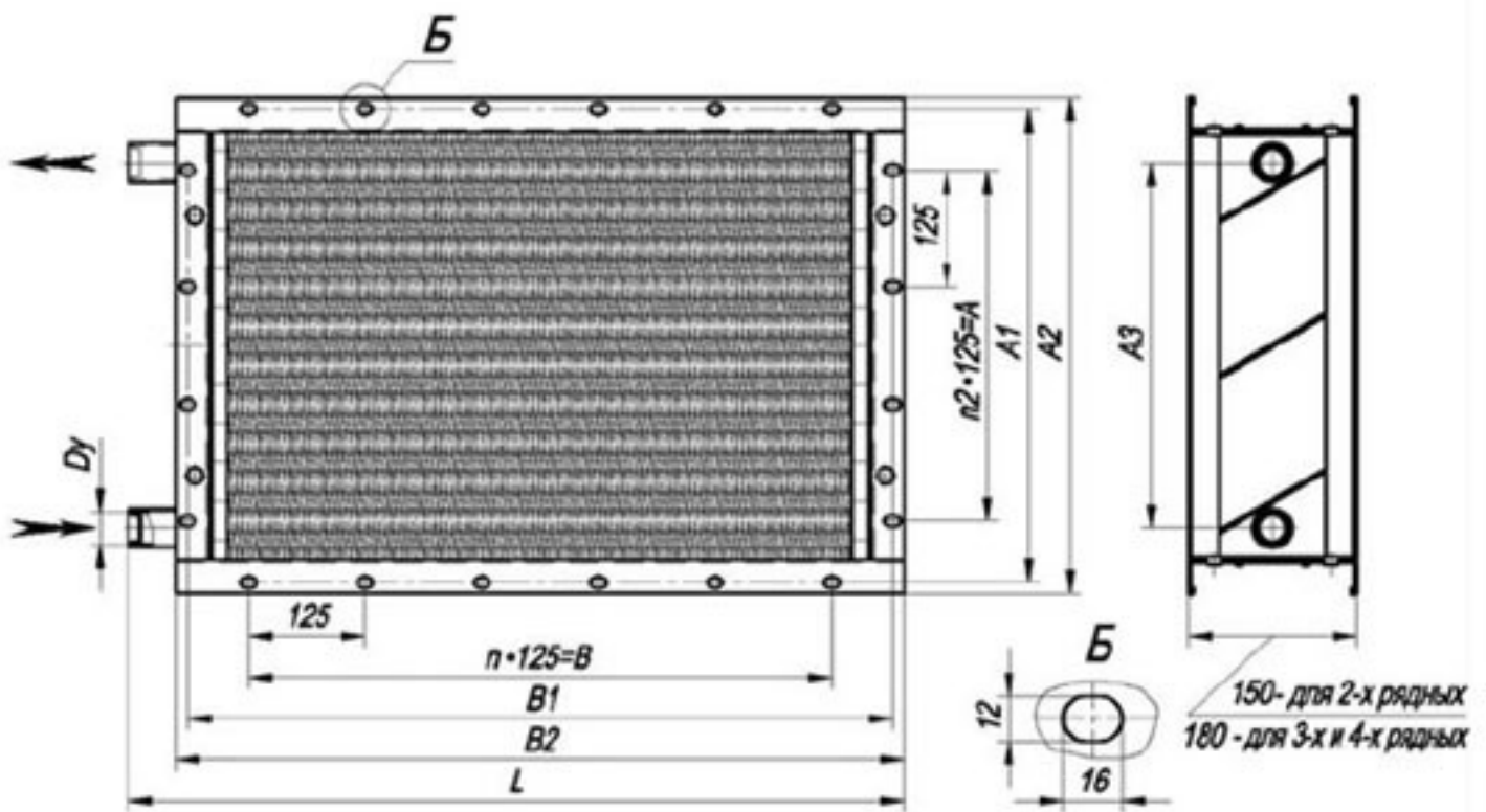
Рис. 1. Калорифер КСк 3-5. Размеры, мм
