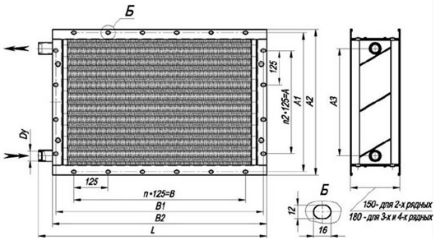
Рисунок 10. Основные размеры, мм
