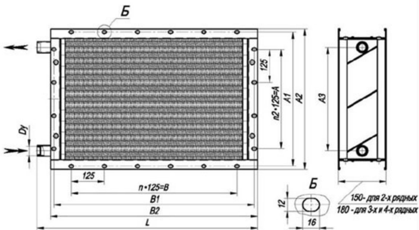
Рисунок 10. Размеры, мм
